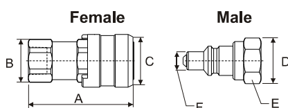
SQB-37
