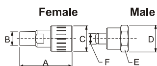
SQB-1/4T
