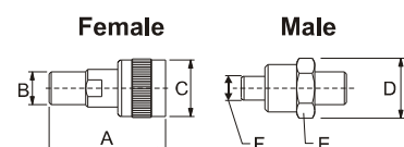
SQB-3/8T
